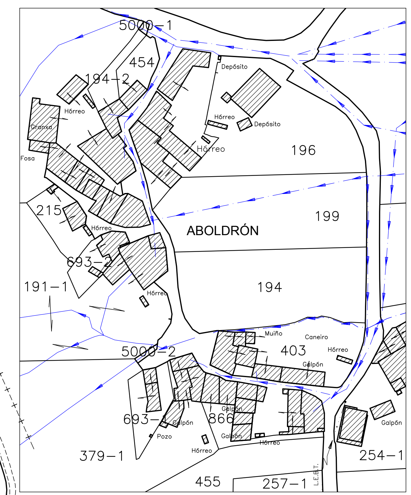
DETALLE ABOLDRÓN 1:1.000
